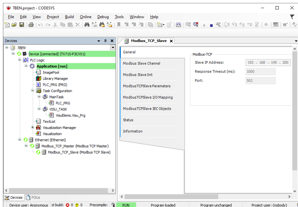
Fig. 65: Modbus TCP communication
