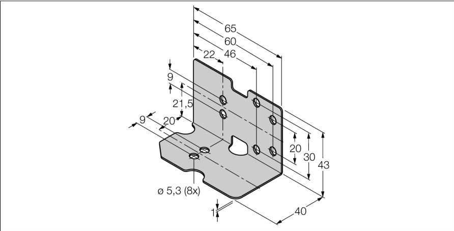
■ 保护框架(L型)
